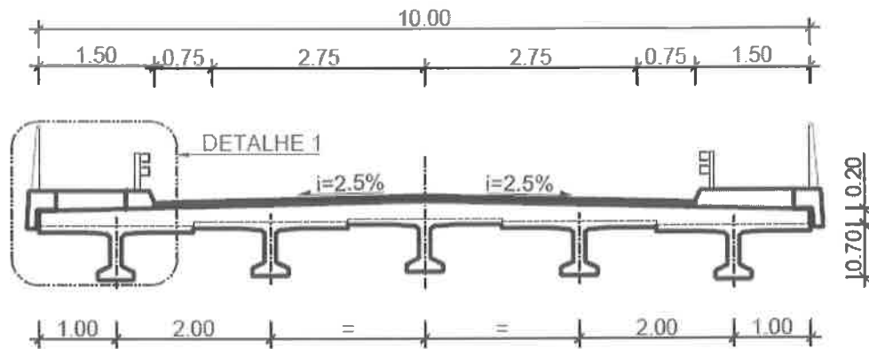
Figura 1 – Corte transversal da Ponte
