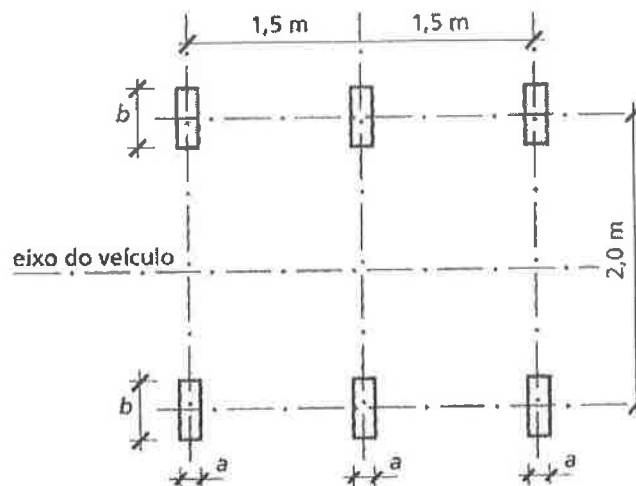
Figura 1 – Veículo tipo considerado
